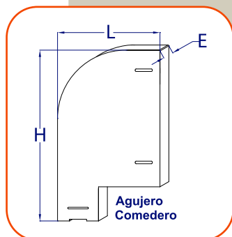
SEPARADOR M3 SB-S1
