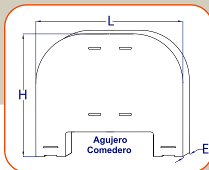
SEPARADOR M3 SB-D1
