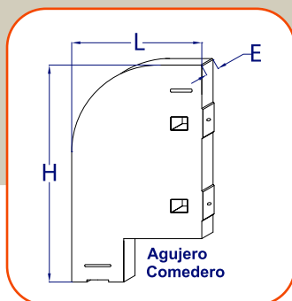
SEPARADOR M3 SB-S2
