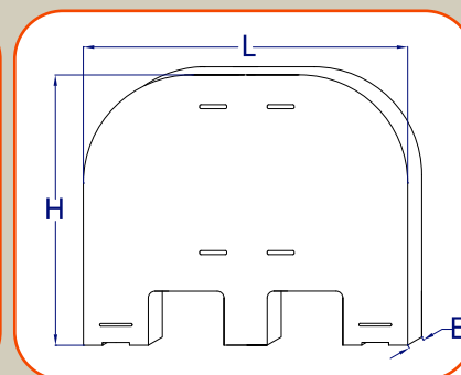
SEPARADOR M3 SB-D2
